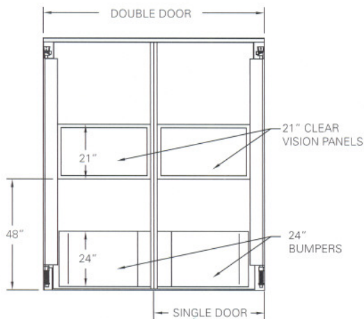
Standard 4800 Door
